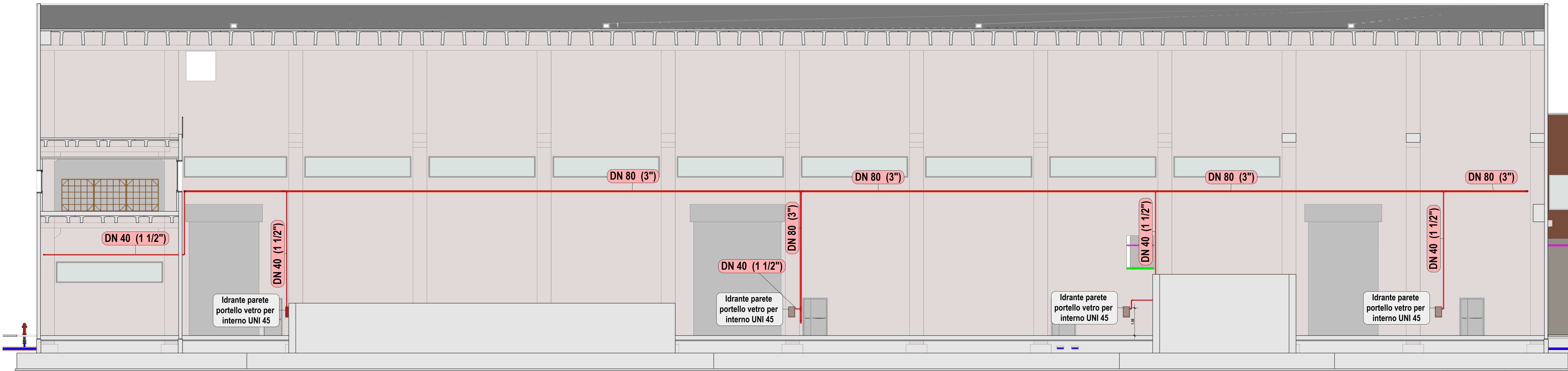
EDIFICIO 1 SEZIONE A-A
