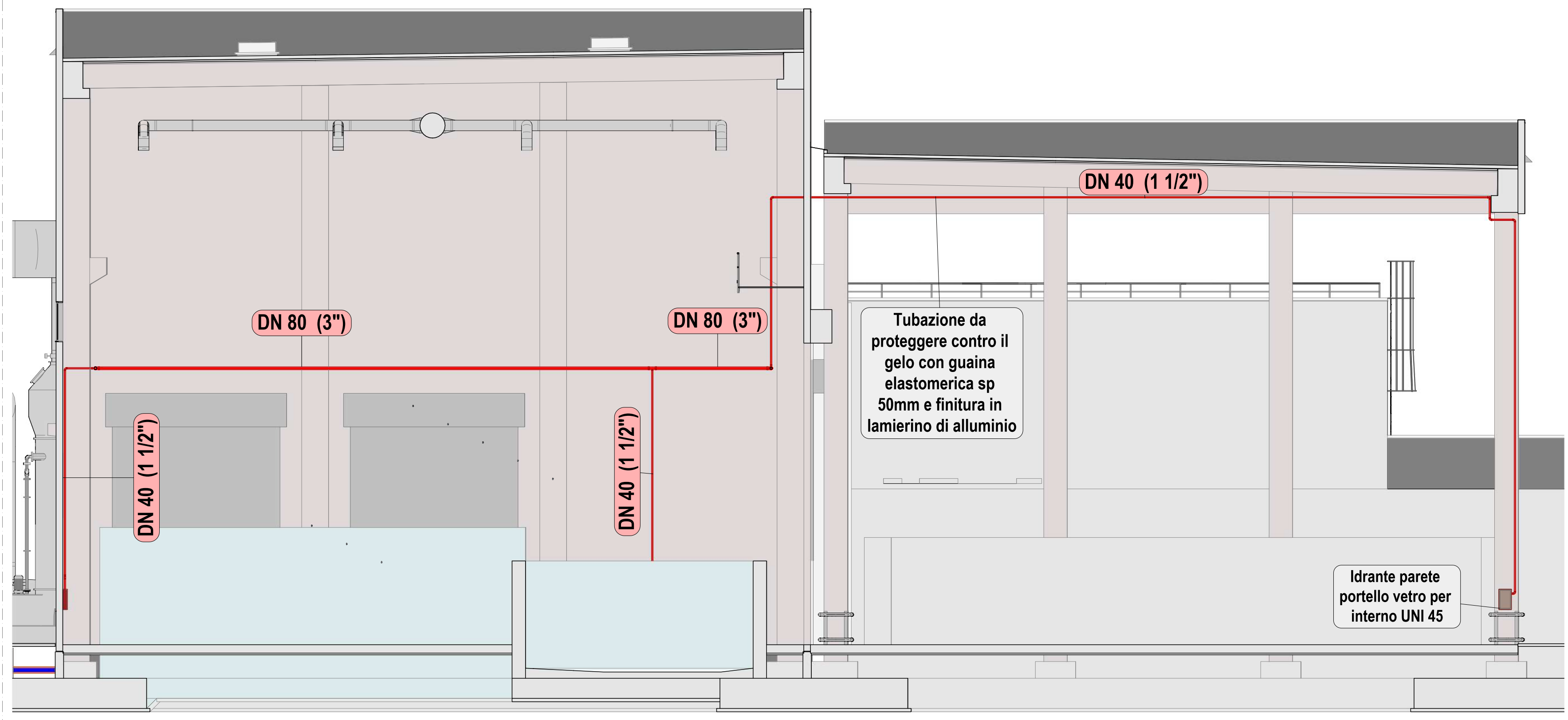
EDIFICIO 1 SEZIONE B-B
